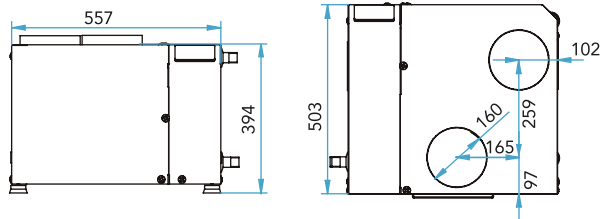
Medidas THX10
