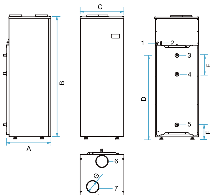
Esquema THP500
