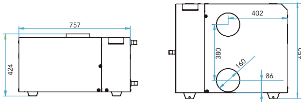
Medidas THX10
