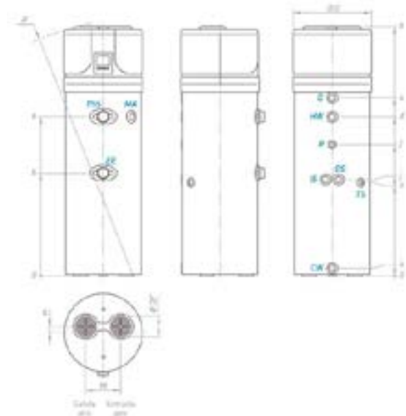
Esquema THP
