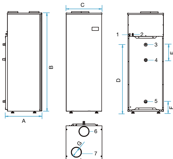
Esquema THP500P
